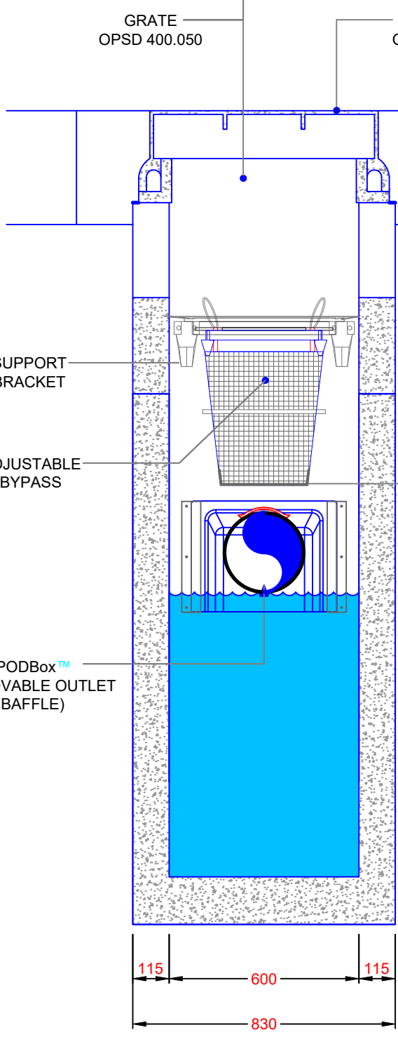
SECTION A-A
