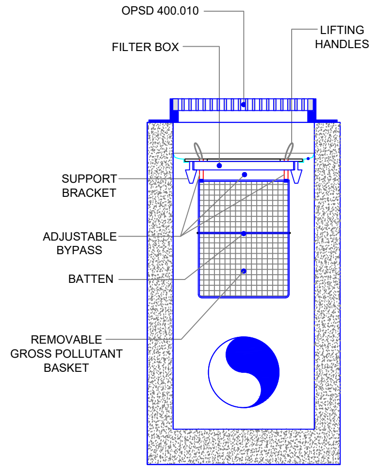
SECTION A-A
